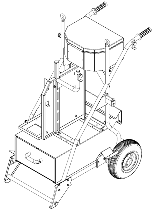
Разгруженная транспортная тележка
