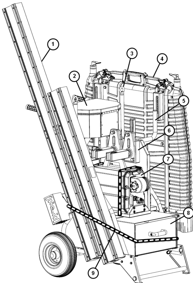
Загруженная транспортировочная тележка, спереди
